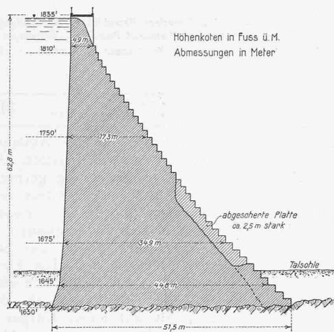
Abb. 5. Rissbildung in dem vollen Strebenaueschnitt der St. Francis-Staumauer entsprechend der Strebenauchung (vergl. „S. B. Z.“ Bd. 91, S. 193, 21. April 1928).
