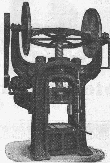
Doppelständerige Exzenterpresse
