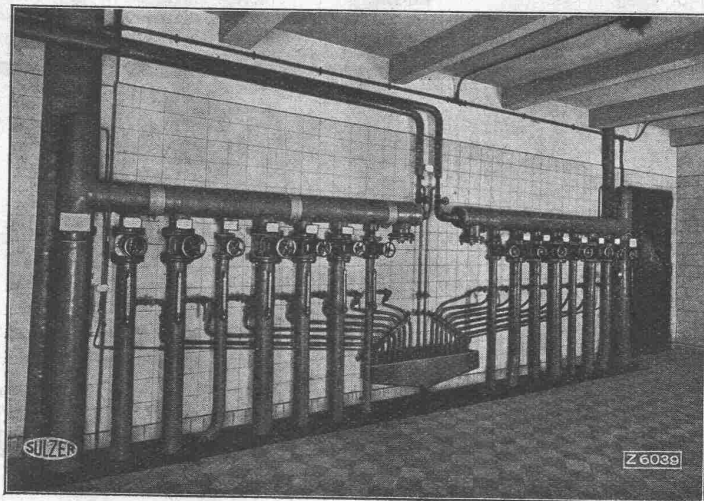
Regulierraum einer Sulzer-Pumpen-Warmwasserheizung
