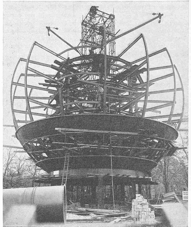
Abb. 1. Eisenkonstruktion der M. A. N., Werk Gustavsburg.
