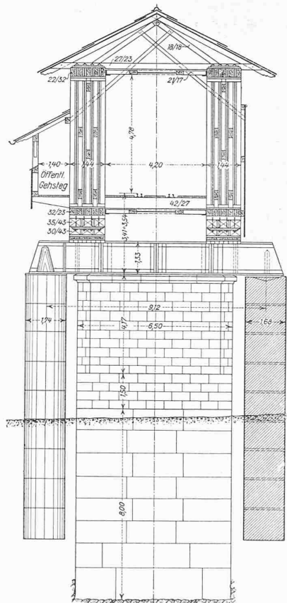
Abb. 3. Querschnitt der Ragazer-Brücke mit Röhren- und Steinpfählen. — 1 : 200.
