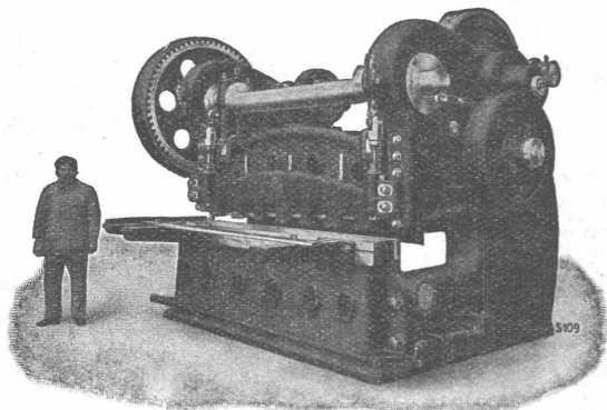
Kurbel-Blechtafelschere
