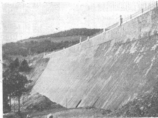
Staumauer Escorial in Spanien, die während des Wasserhochstandes mit schnellbindender „SIKA“ gedichtet wurde.
