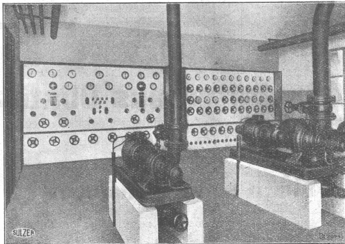
einer Sulzer-Warmwasserheizung in einer Grossbank
