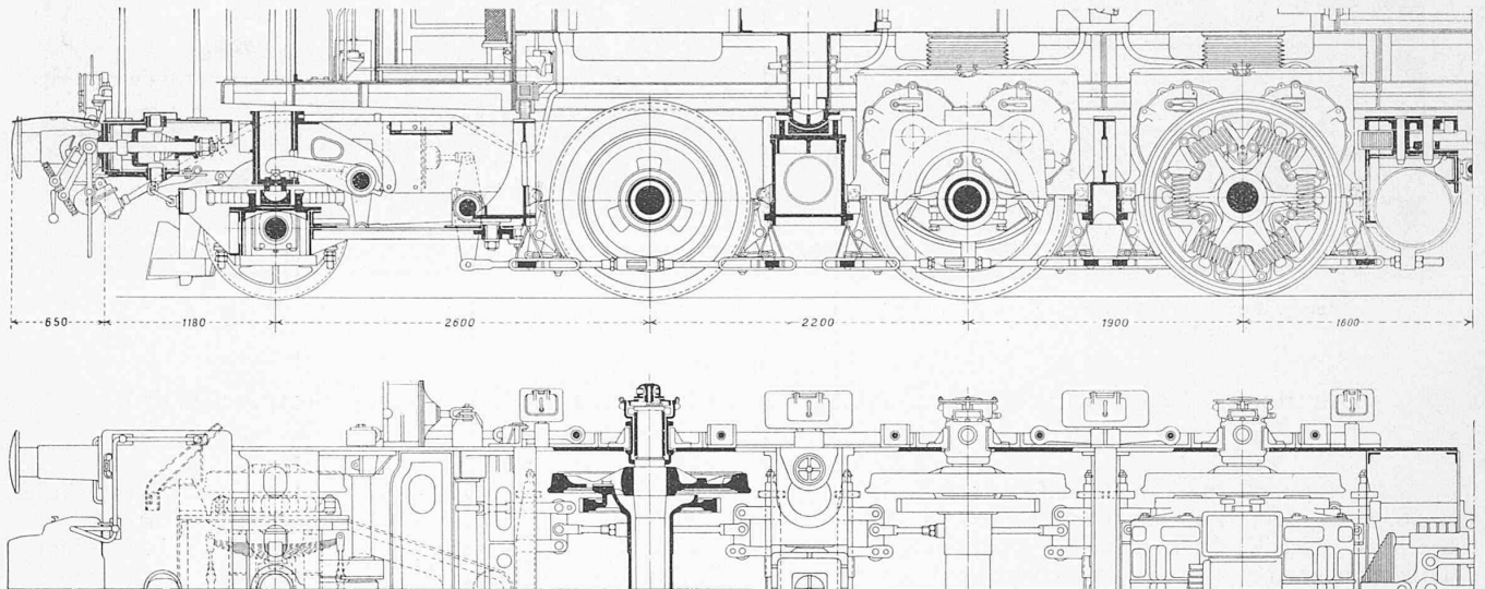
Abb. 5. Längsschnitt durch ein Drehgestell, sowie Draufsicht mit Schnitt durch den Hohlwellen-Antrieb. — Masstab 1 : 50.
