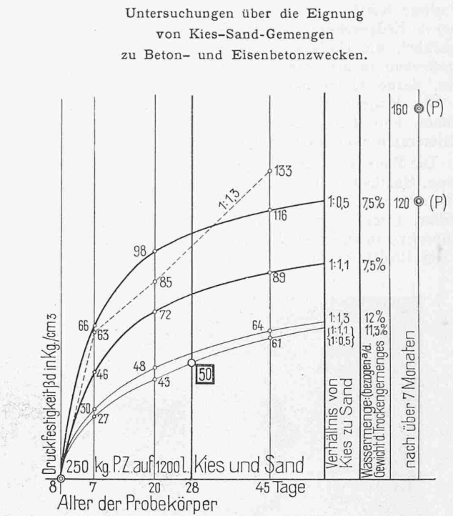
Abb. 4 und 5. Erhärtungskurven des Beton, hergestellt aus dem Kies-Sand-Gemenge E, links mit 300 kg, rechts mit 250 kg Portland-Zement auf 1200 l Kies und Sand. — — — Erhärtungskurven für plastischen Beton unter Verwendung von Zement II (Normenfestigkeit 359 kg/cm 2 ). — — — Erhärtungskurven für Gussbeton unter Verwendung von Zement II. — — — Erhärtungskurven für plastischen bzw. Gussbeton unter Verwendung von Zement III (Normenfestigkeit 710 kg/cm 2 ). Die mit A und P bezeichneten Punkte sind Kontrollversuche, erhalten aus der Probebelastung (P) oder ermittelt an ausgespitzten Betonkörpern (A).
