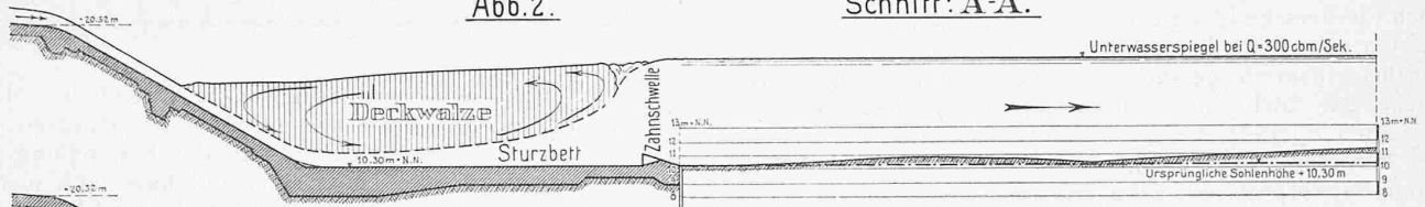
Schnitt: A-A.
