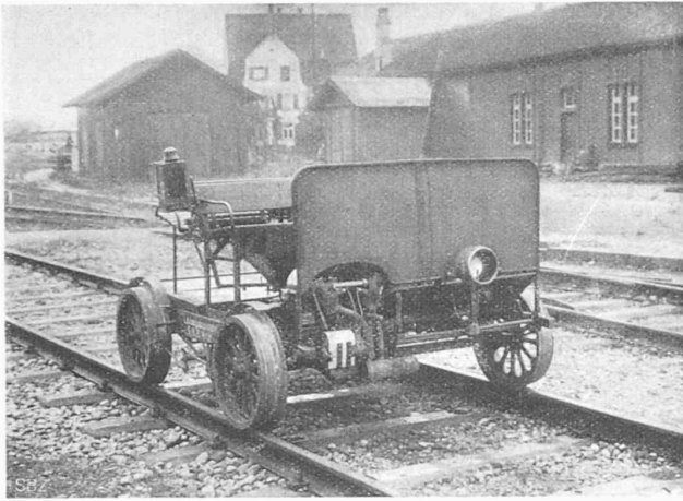
Abb. 3. Motor-Draisine des Leitungsaufsehers.
