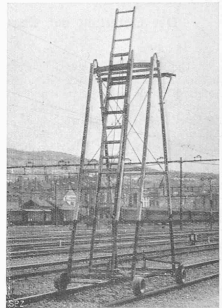
Abb. 4. Roll-Leiter für Fahrleitungs-Montage.
