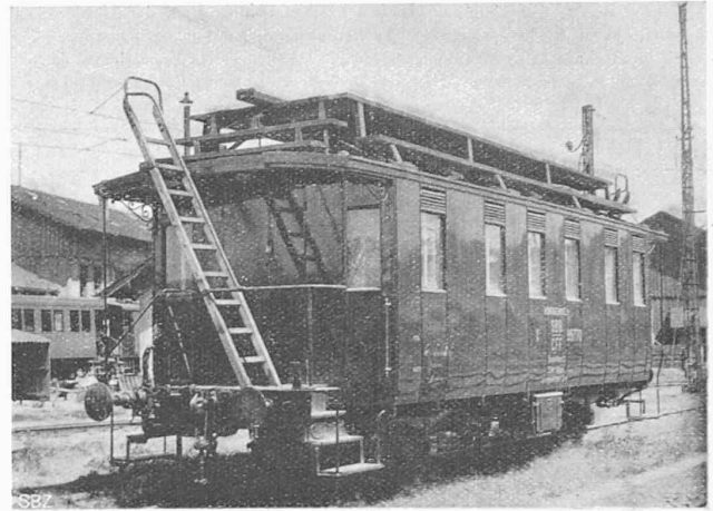
Abb. 5. Reparaturwagen für Fahrleitungs-Anlagen.
