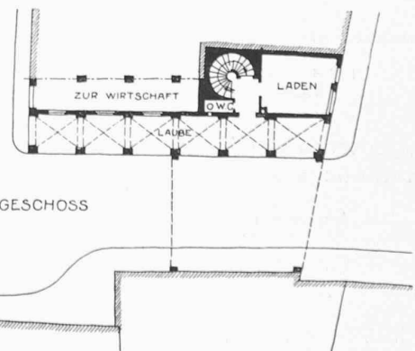
Umbau des Tors II und des Hauses Rohr. — Grundrisse 1:400.
