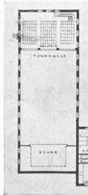
Grundrisse vom Erdgeschoss und Obergeschoss. Masstab 1:800.
