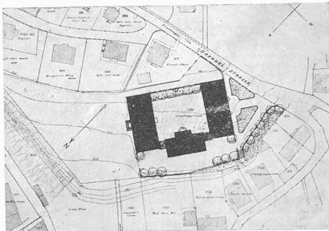
Lageplan. — Masstab 1:2000.
