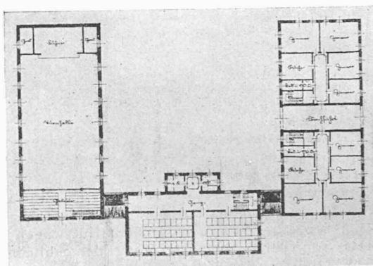
Grundriss vom Obergeschoss.
