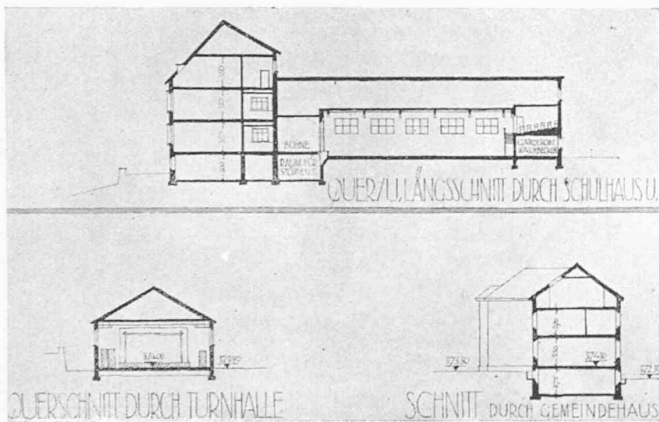
Schnitte. — Masstab 1: 800.
