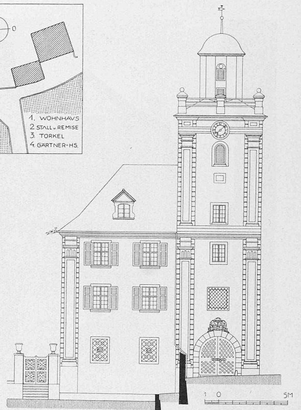
Ostfassade nach dem Umbau
