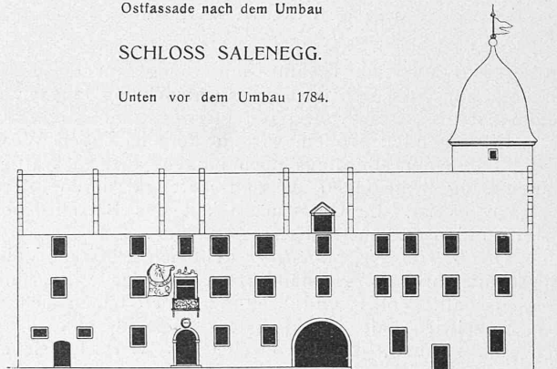
Ostfassade nach dem Umbau
