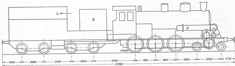
Abb. 7. Lokomotive von Zoelly mit Dampfturbinen-Antrieb, gebaut 1920 von Escher Wyss & Cie., Zürich. Masstab 1 : 150. — A Abdampfrohr, B Kohlen und Wasser, L Luftkanal, T Dampfturbine.
