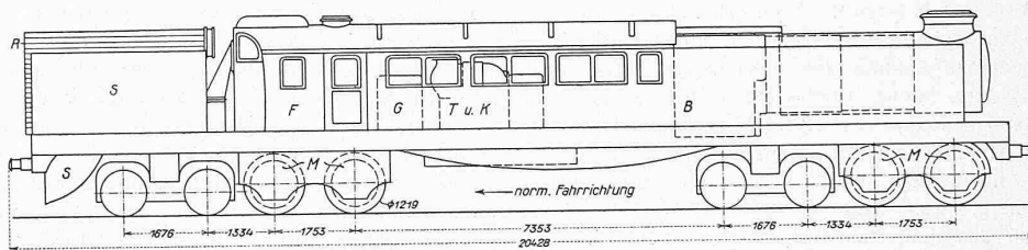
Abb. 4. Lokomotive von Reid und Ramsay mit turbo-elektrischem Antrieb. — Masstab 1 : 150. B Kohlen und Wasser, F Führerstand, G Generator, T Turbine, K Kondensator, M Motoren, S Luffträger, R Rohrbündel.
