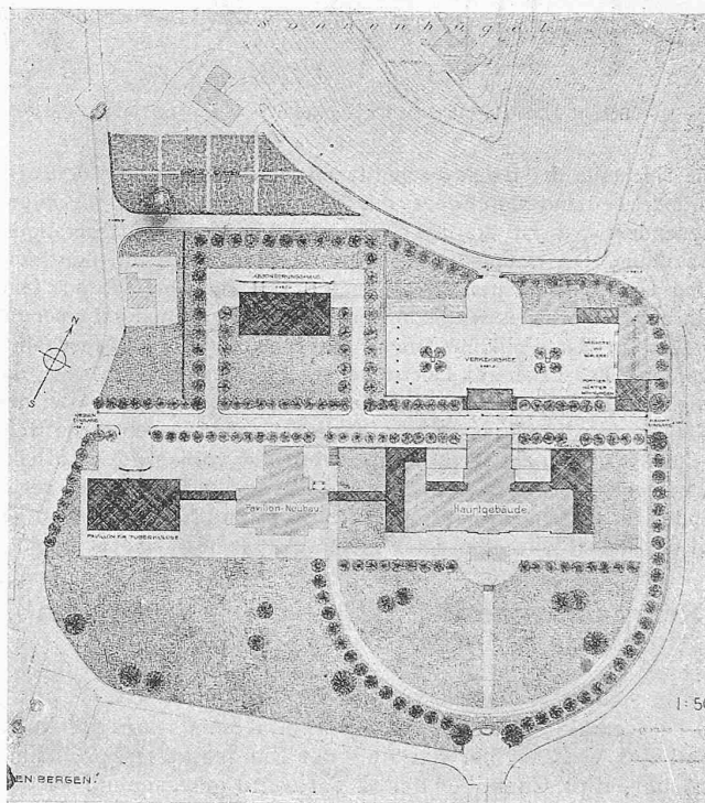
I. Rang ex aequo, Entwurf Nr. 7. Lageplan 1:2500. Verfasser: Arch. H. Leuzinger (Glarus) und P. Truniger (Wil).
