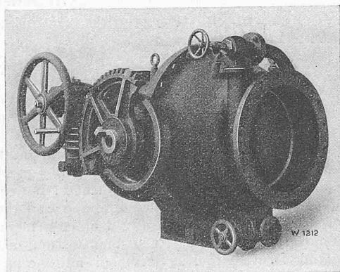
Abb. 5. Ansicht des EWC-Kugelschiebers.
