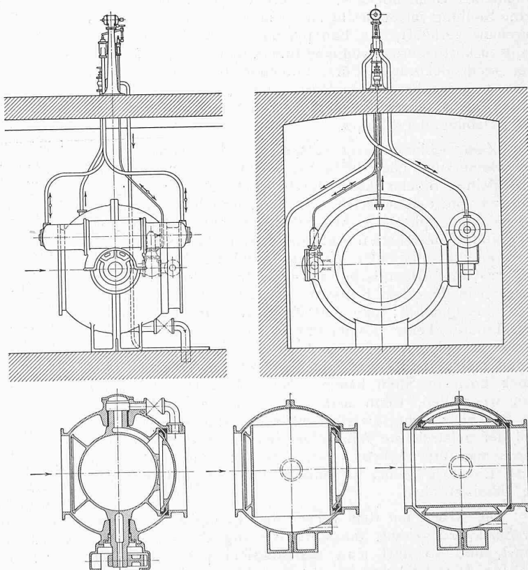
Abb. 4. Ansichten, Horizontalschnitte und Vertikalschnitte des EWC-Kugelschiebers.
