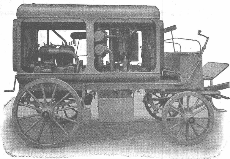
Fahrbare Kompressor-Anlage
