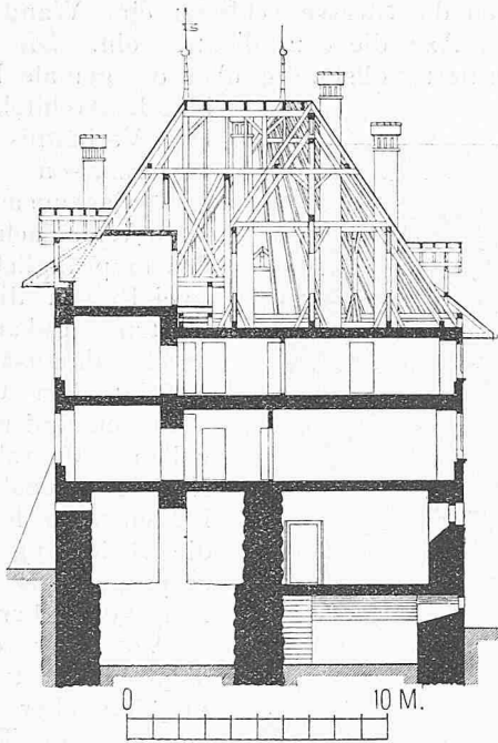
Schnitt. — Masstab 1 : 300.
