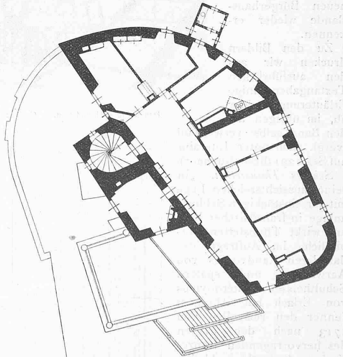
Grundriss des zweiten Stockwerks, Masstab 1 : 300.
