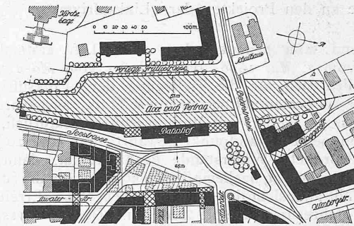
Abb. 3. Erweiterungs-Vorschlag Hochbauteam 1914.
