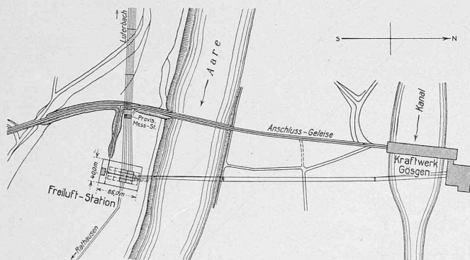
Abb. 3. Situationsplan der Freiluft-Schaltstation Gösigen. — Masstab 1 : 8000.
