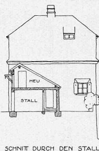
Angekaufter Entwurf Nr. 4. Arch. J. U. Könz in Guarda. Einheitl. Masstab 1:300.
