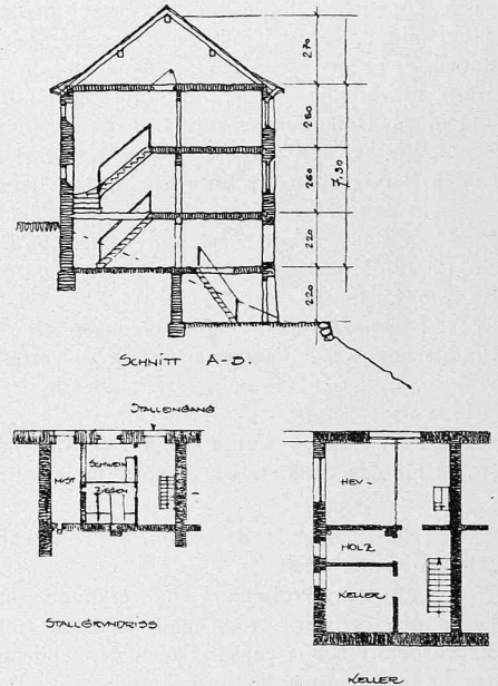
Angekaufter Entwurf Nr. 9. — Verfasser Arch. Enrico Bisaz in Zerne. — Masstab 1:300.
