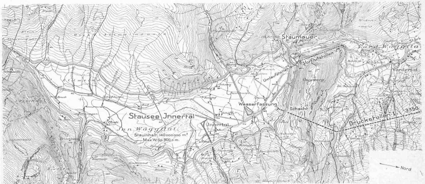
Abb. 6. Kraftwerk Wäggitel: Stausee im Innerthal mit Staumauer, Wasserfassung und Druckstollen I. — Masstab 1:35 000 (10 m-Kurven).
