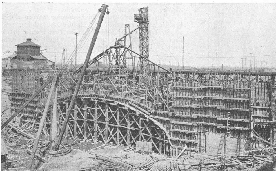
Abb. 42. Schalung und Betonier-Einrichtung für eine Bahnüberführung über den Kanal.
