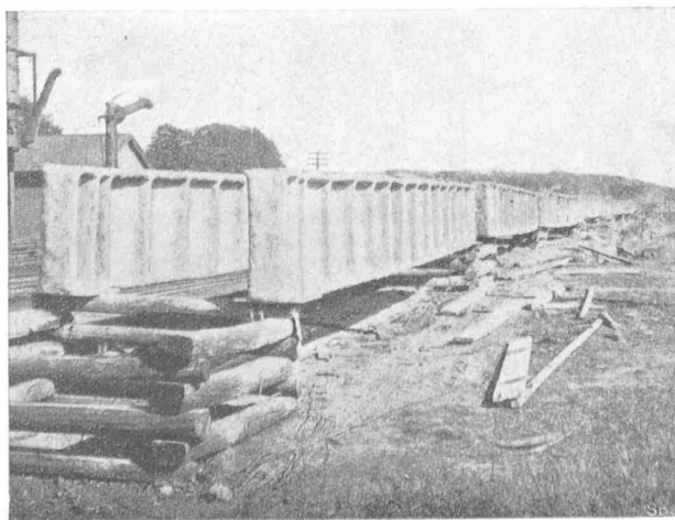
Abb. 4. Blechbalken-Brückenträger mit Rostschutz-Ueberzug aus „Guniting“ auf Drahtgeflecht, bei Worcester Mass.
