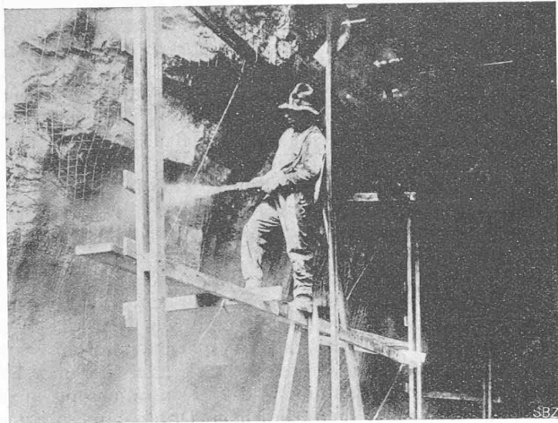
Abb. 7. „Guniting“-Schutzverkleidung gegen Abwitterung in einem unausgemauerten Tunnel der Illinois Central Ry.
