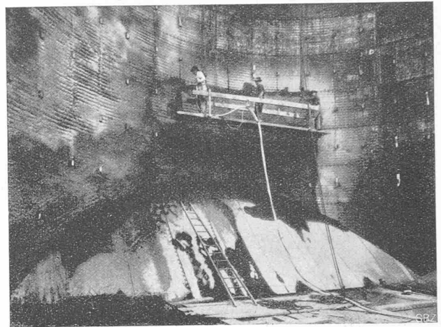
Abb. 5. Kohlsilo aus Stahlblech mit 5000 t Fassungsraum wird inwendig mit „Guniting“ auf Drahtgeflecht überzogen.
