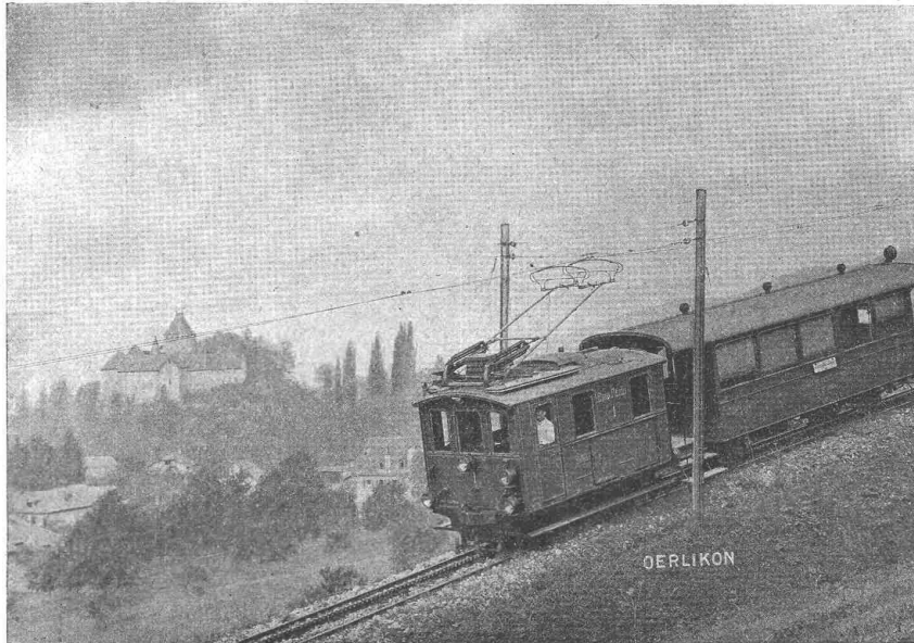
Elektrische Zahnradbahn Blonay-les Pléiades (s. Vevey)
