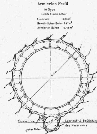
Abb. 12. Armiertes Profil.
