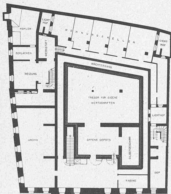
Abb. 1. Keller-Grundriss.
