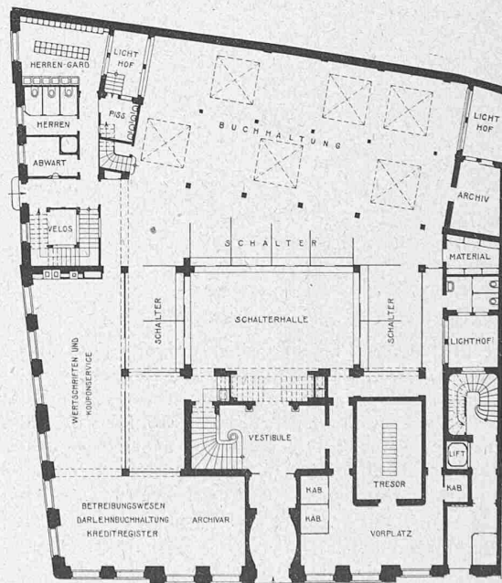
Abb. 2. Erdgeschoss 1: 400.
