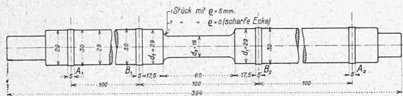
Abb. 1. Probestäbe für die erste Versuchsreihe.
