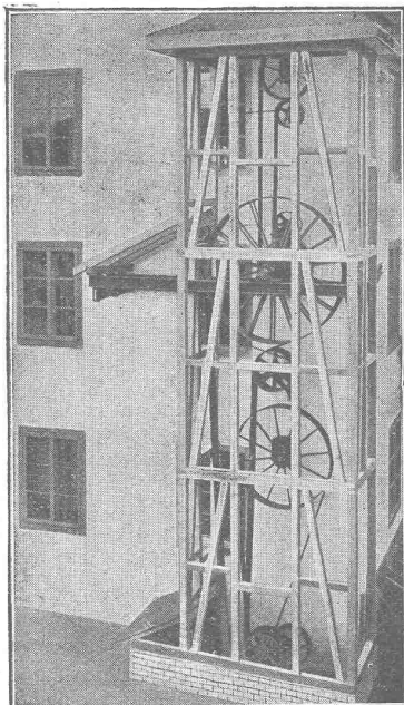
Umänderung einer stehenden Welle mit konischen Rädern in vertikale Lenix- Riementreibe in einer Baumwollweberel
