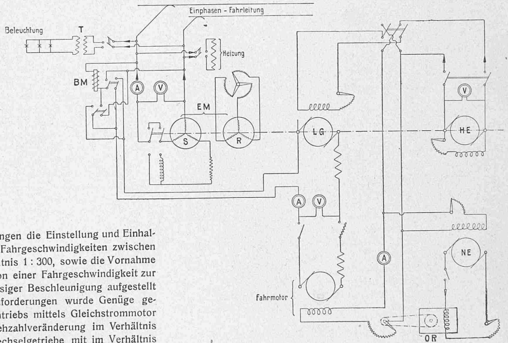
Abb. 4. Schaltungsschema.
