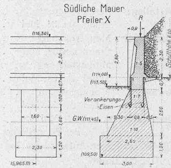
Abb. 3. Ansicht und Schnitt. Masstab 1:200.
