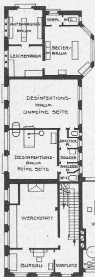
Abb. 9 bis 12: Grundrisse 1:400 von beiden Kellergeschossen, Erdgeschoss und Obergeschoss.
