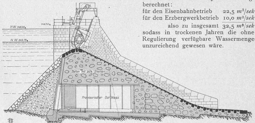
Abb. 3. Schnitt durch die Flossgasse und den prov. Grundablass. — Masstab 1:300.
