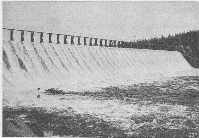
Abb. 5. Ansicht des Ueberfall-Wehres.
