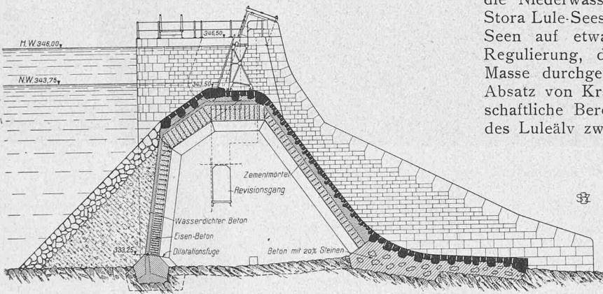
Abb. 4. Schnitt durch das Ueberfallwehre. — Masstab 1:300.
