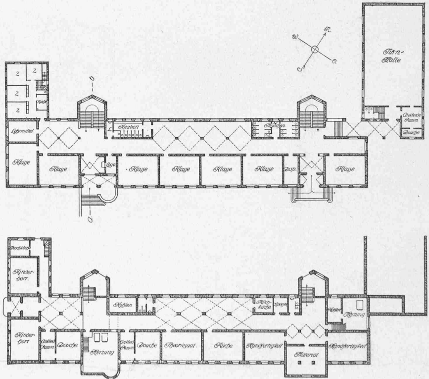
3. Rang. Entwurf Nr. 37. „Hutten“. — Grundrisse und Schnitt a-b. — Masstab 1 : 800.
