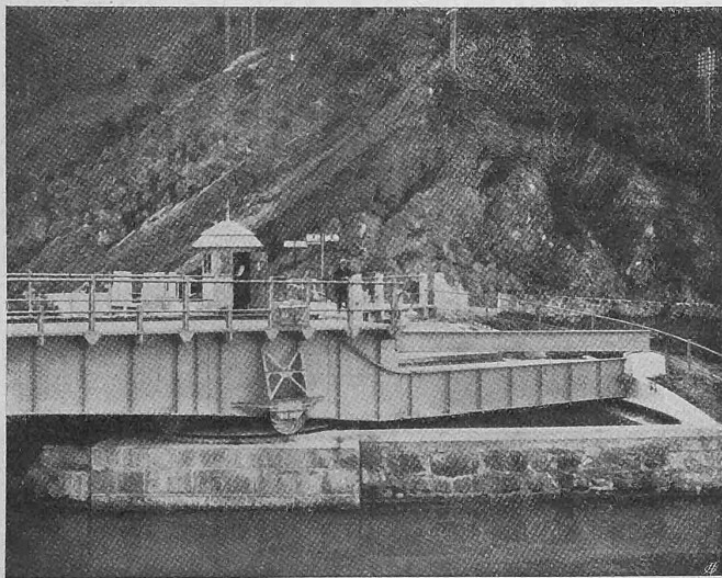
Abb 15. Widerlager und Gegengewichtsarm der Drehbrücke, in halbgeöffneter Lage, vom festen Brückenende aus gesehen.
