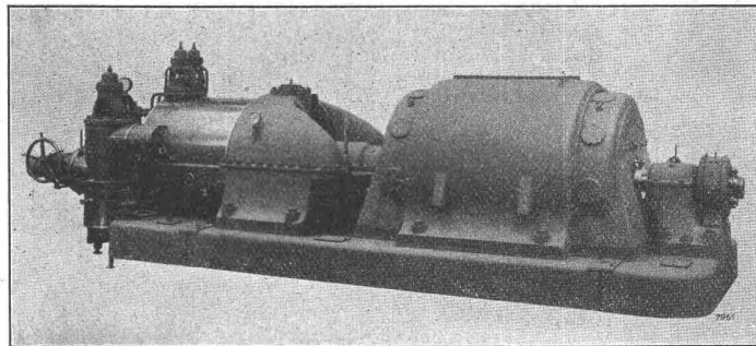
Drenstrom-Turboaggregat, Normalleistung 5000 kW, 3000 Umdr./Min.
