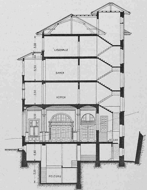
Abb. 11. Schnitt durch den Speisesaal. — 1:300.
