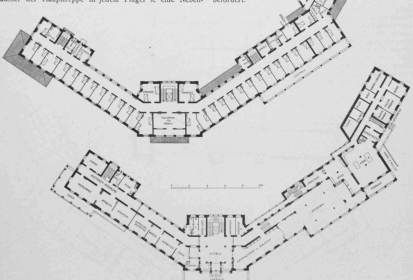
Abb. 7 und 8. Grundrisse vom Erdgeschoss und I. Stock (Herren-Abteilung). — Masstab 1:600.
