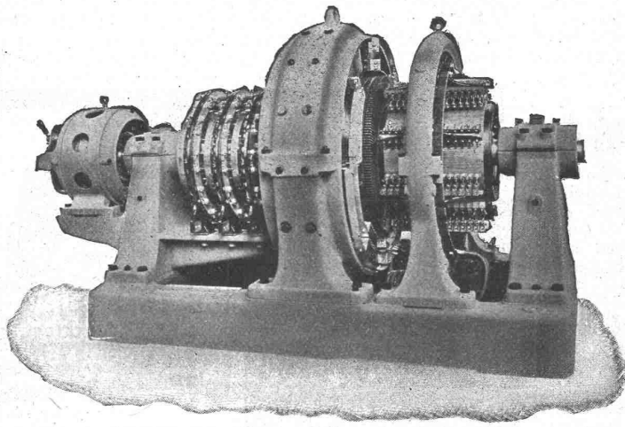
Einanker-Umformer.
