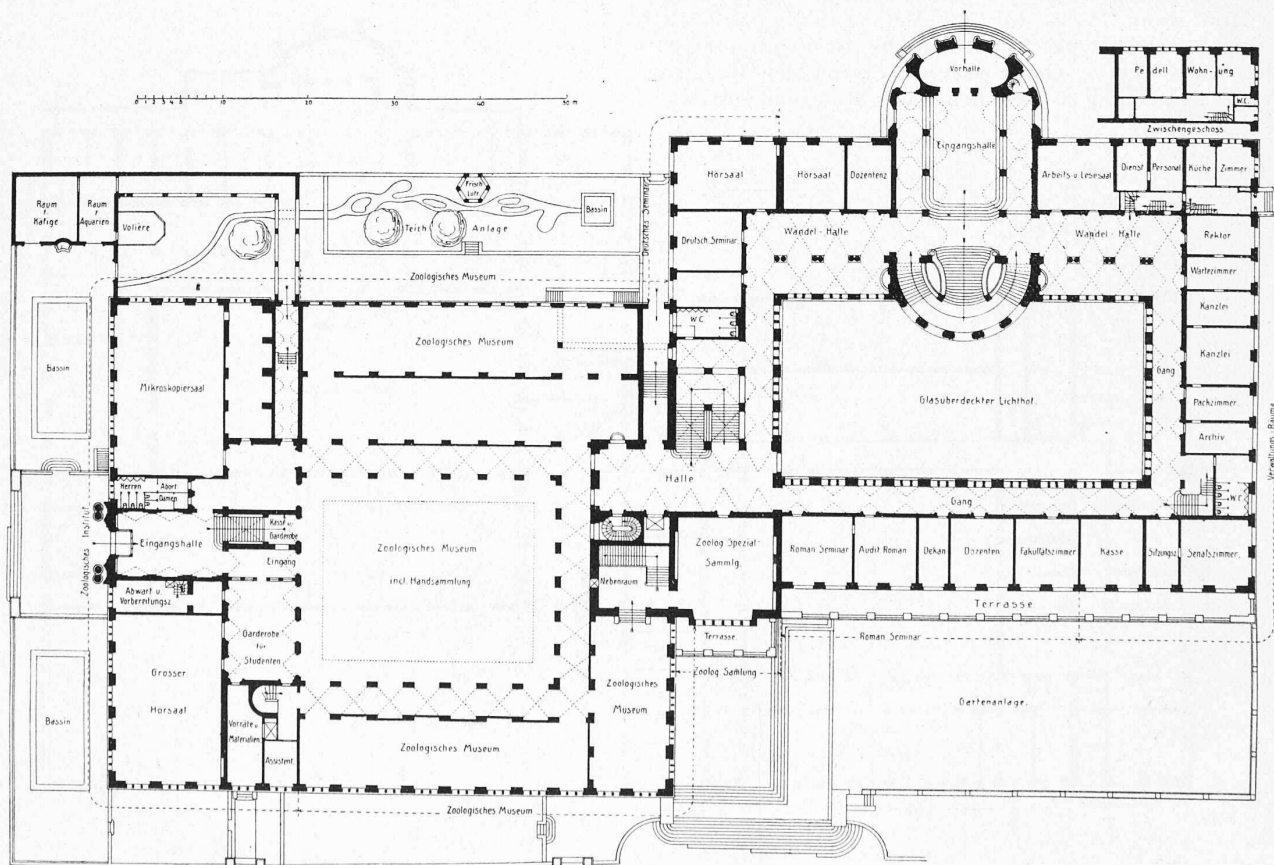
Abb. 11. Grundriss vom Erdgeschoss. — Masstab 1:800.
