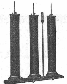
Wasserwiderstand
