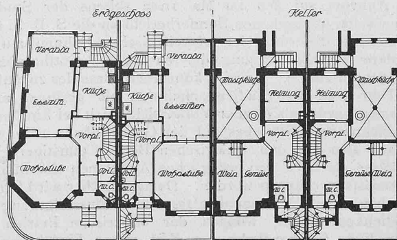
Abb. 1. Gesamtbild vom Parkweg aus. — Abb. 2 bis 5. Grundrisse 1:400.
