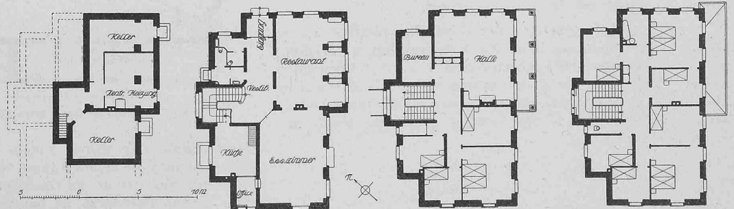
Abb. 5 bis 8. Grundrisse.
