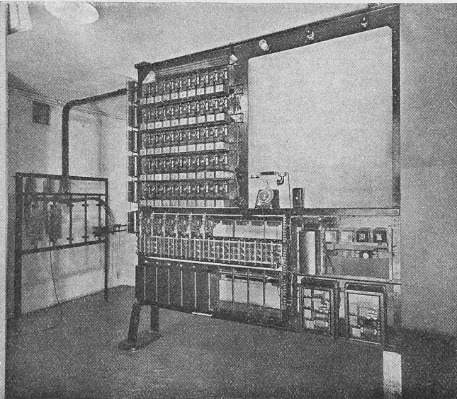
Abb. 9. Automatische Telephonzentrale.
