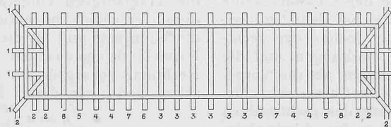
Abb. 10. Holzschwellenlager eines Caissons.
