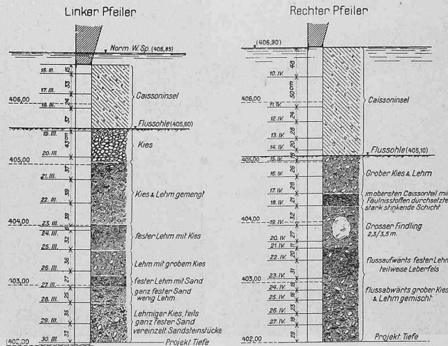
Abb. 6. Beschaffenheit des Baugrundes. — 1 : 80.
