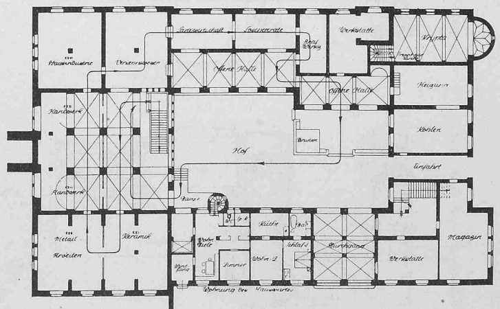
I. Preis. „An stillen Wassern“. — Grundrisse vom Unter- und Erdgeschoss 1:600.
