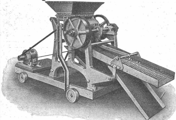
Fahrbarer Koksbrecher mit elektrischem Antrieb.
