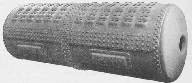
Abb. 16. Garbe-Unterkessel.
