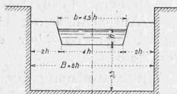
Abb. 12. Ueberfall Cipolletti.
