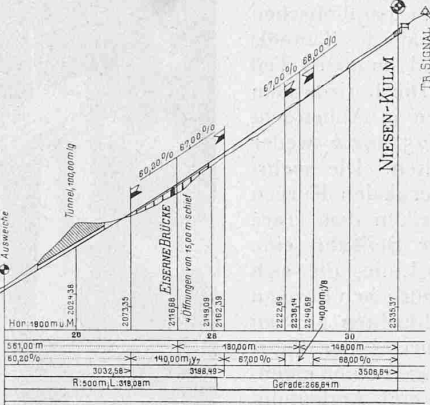
Abb. 5. Längsprofil der II. Sektion.
